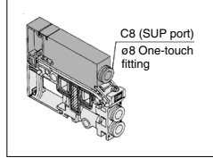
Individual SUP spacer VVQ2000-P-1- C8 / N8
